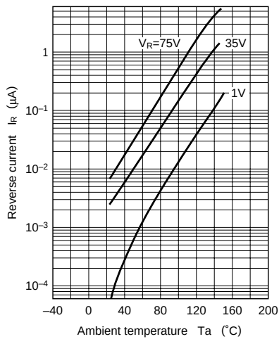
I_R - T_a
