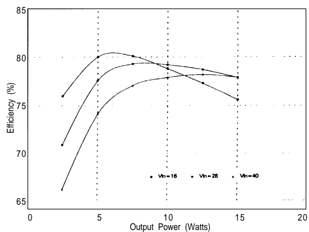
ATO2815T EFFICIENCY
