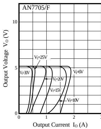
V_O - I_O
