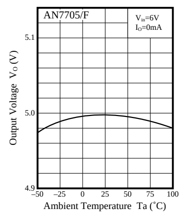
V_O - T_a
