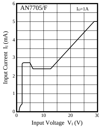
I_I - V_I
