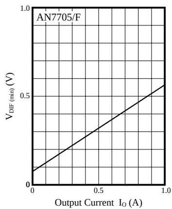
V_{DIF}(\text{min}) - I_O
