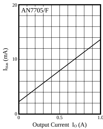
I_{bias} - I_O
