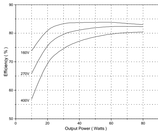
AFL27005S
