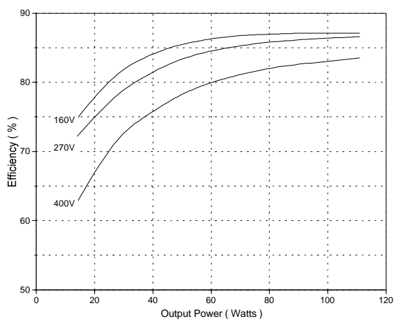
AFL27028S
