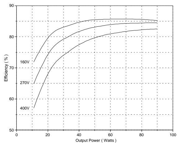
AFL27009S
