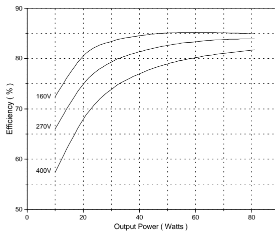
AFL27006S
