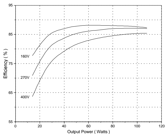
AFL27012S
