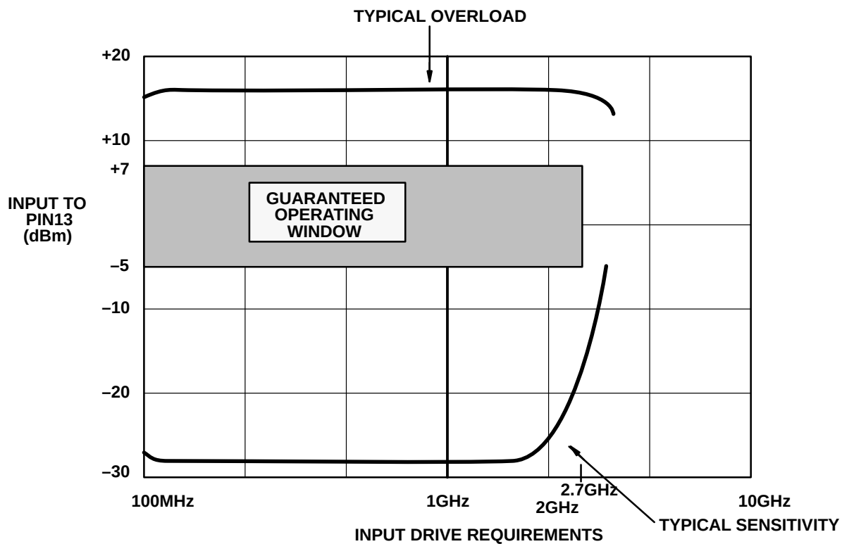
Fig. 3 SP8852E
