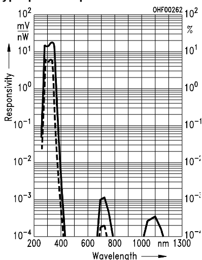
Fig. 1 Typ. spektr. Verhalten des UV Sensors Typ. spectr. response of the UV sensor
