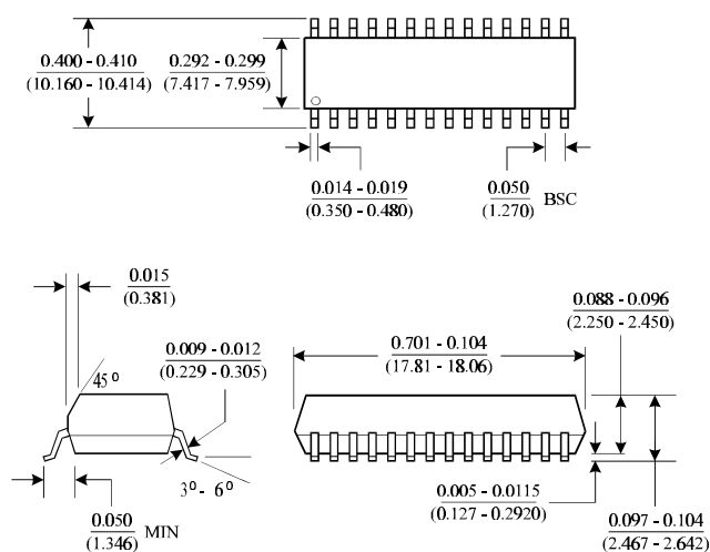
28 PIN SOIC
