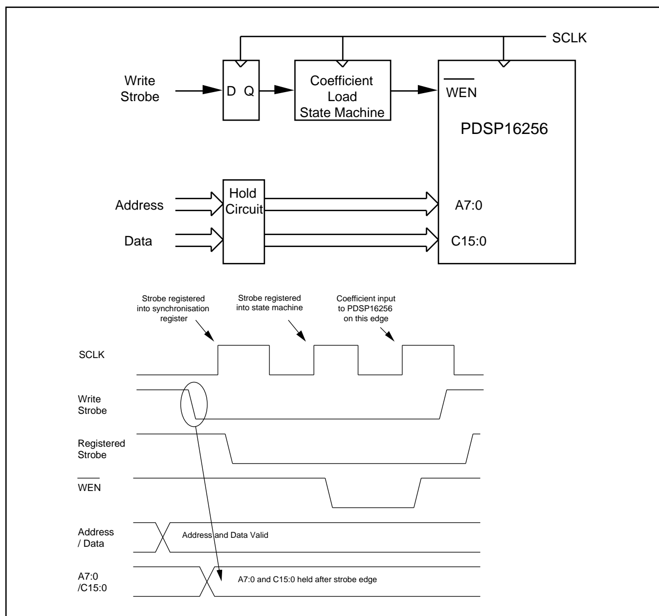
Fig. 18 Remote Master Synchronisation
