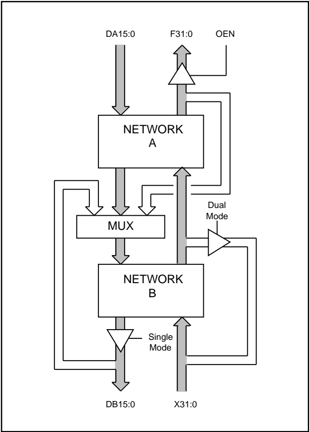
Fig. 6 Single Filter Bus Utilisation
