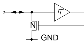
Fig. 8-11: Input/Output Pins 8 and 9 (I 2 C_DA, I 2 C_CL)
