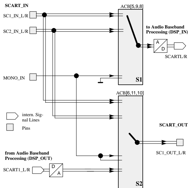
Fig. 4–3: SCART-Switching Facilities (s. 7.3.17.)
