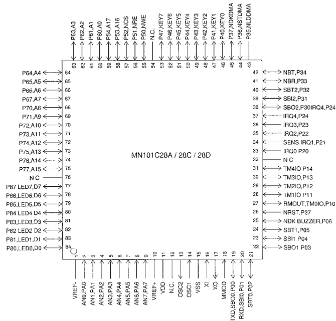
QFP084-P-1818E
