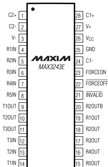
SO/SSOP
