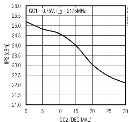
IIP2 vs. GC2
