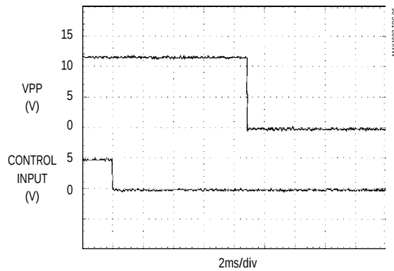
VPP SWITCHING (FALL)
