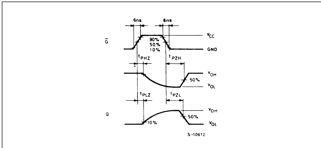
WAVEFORM 9 : ( f=1\text{MHz} ; 50% duty cycle)
