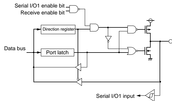
(6) Port P4 4
