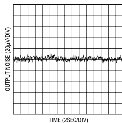
Output Noise 0.1\text{Hz} \leq f \leq 10\text{Hz}
