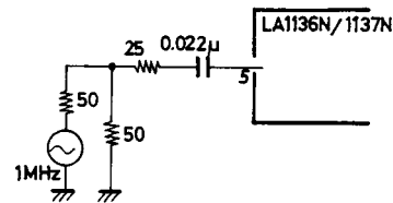
Mixer input
