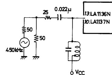
Detector input
