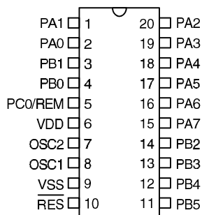
HT48RA0 - 20 SOP-A
