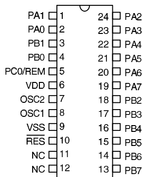
HT48RA0 - 24 SOP-A
