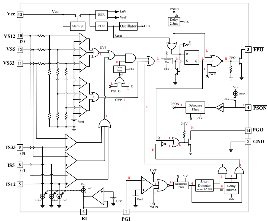
FAN7685 (FAN7686)
