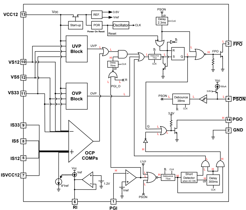
FAN7687
