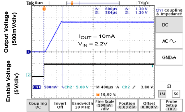
Enable Delay
