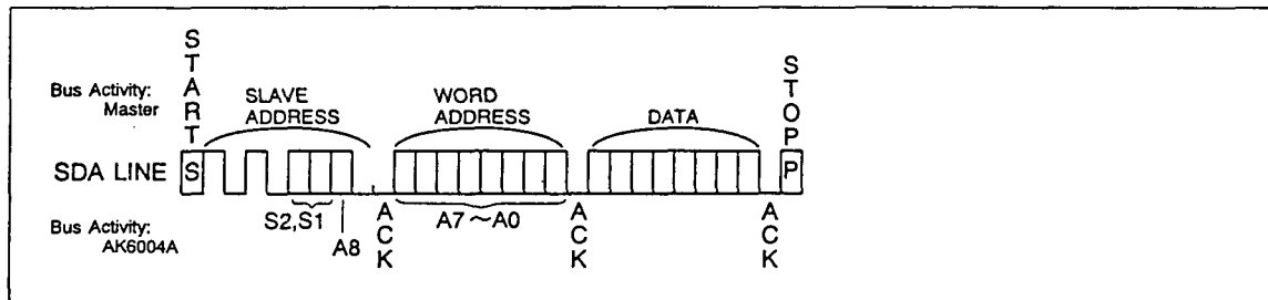
BYTE WRITE
