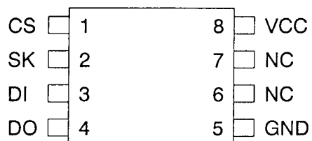
8pinTSSOP
