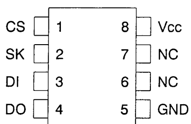
8pinSOP
