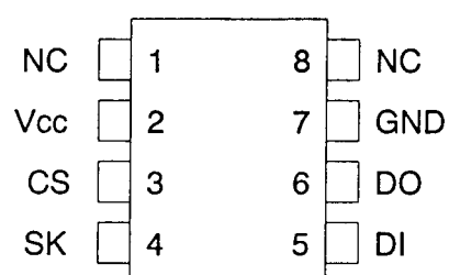
8pinSOP
