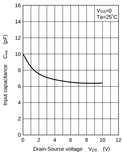
C_{iss} - V_{DS}
