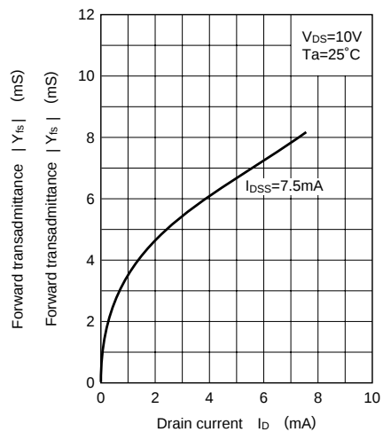
|Y_{fs}| - I_D
