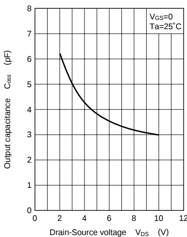
C_{oss} - V_{DS}
