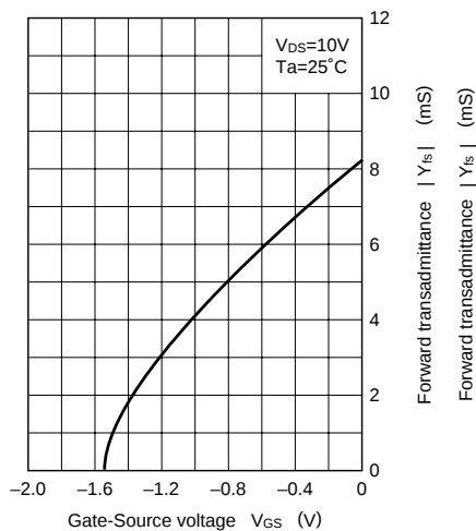
|Y_{fs}| - V_{GS}
