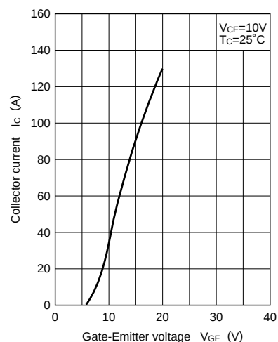
I_C - V_{GE}
