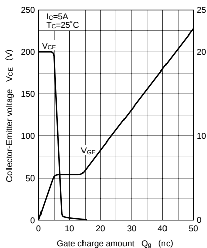
V_{CE}, V_{GE} - Q_g
