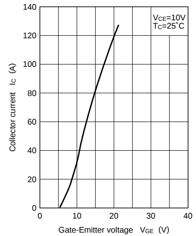
I_C - V_{GE}
