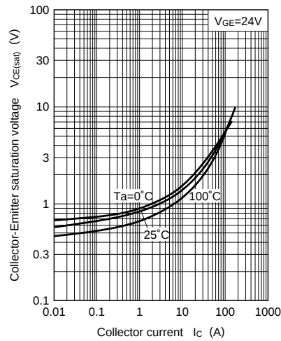
V_{CE(sat)} - I_C
