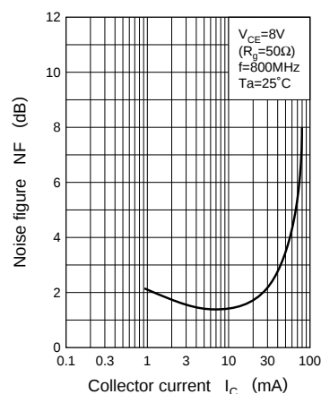
\text{NF} - I_C
