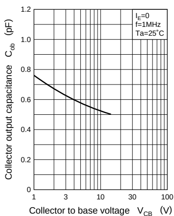
C_{ob} - V_{CE}
