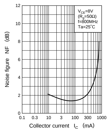
\text{NF} - I_C
