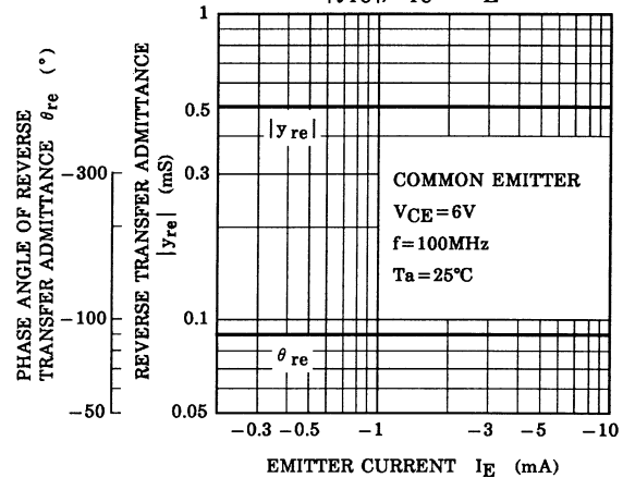
|y_{re}|, \theta_{re} - I_E
