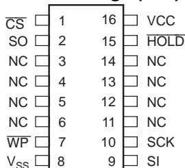
SOIC Package (S16)
