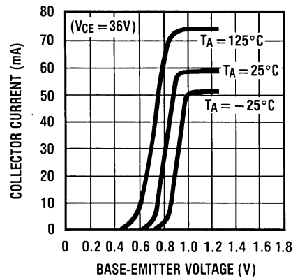
36 Volt Transfer Function
