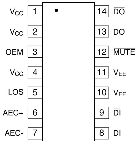
14-Pin SOIC
