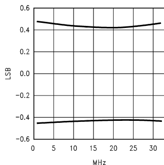
INL vs f_{CLK}
