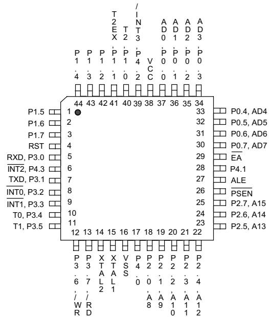
44-Pin QFP/TQFP (W78E58F/W78E58M)
