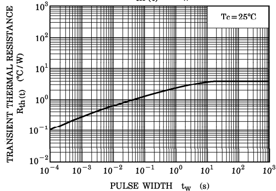
R_{th}(t) - t_w
