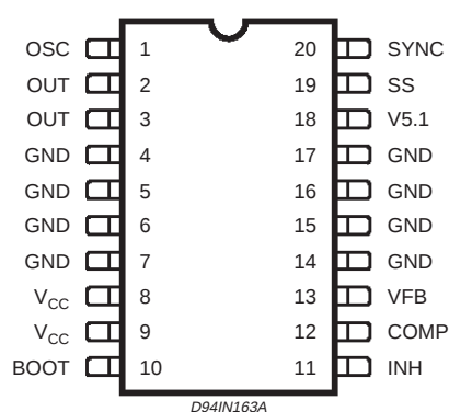
SO20 (12+4+4)
