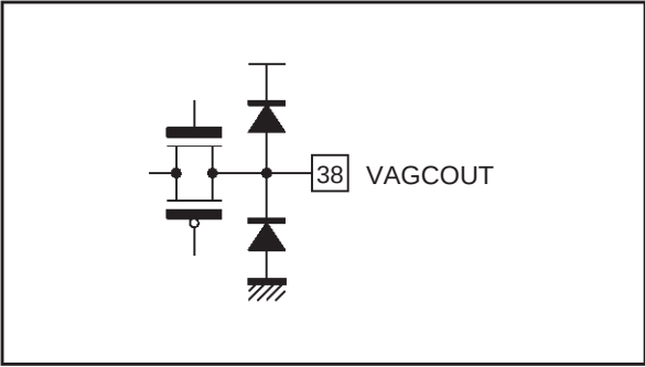
Figure 23 : VAGCOUT
