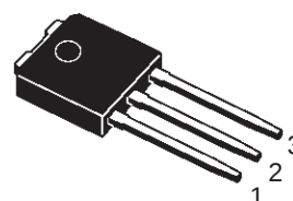
DPAK TO-251 (Suffix "T4")
