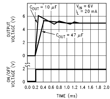
Enable Transient
