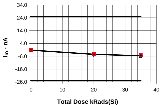
I_{IO} ; V_O=1.5V , COMP 4 vs Total Dose
