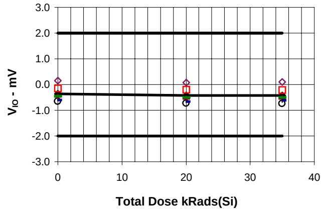
V_{IO} ; V_{+}=30V , COMP 2 vs Total Dose
