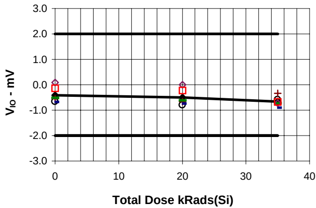
V_{IO} ; V_{CM}=28.5V , COMP 2 vs Total Dose
