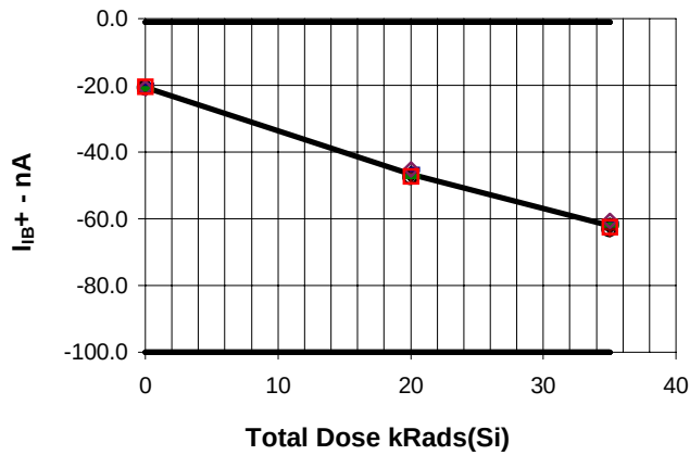
I_{B+} ; V_O=1.5V , COMP 4 vs Total Dose
