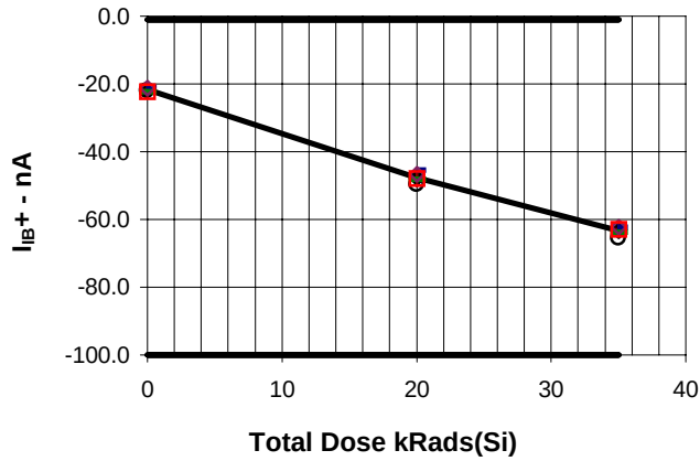
I_{B+} ; V_O=1.5V , COMP 3 vs Total Dose
