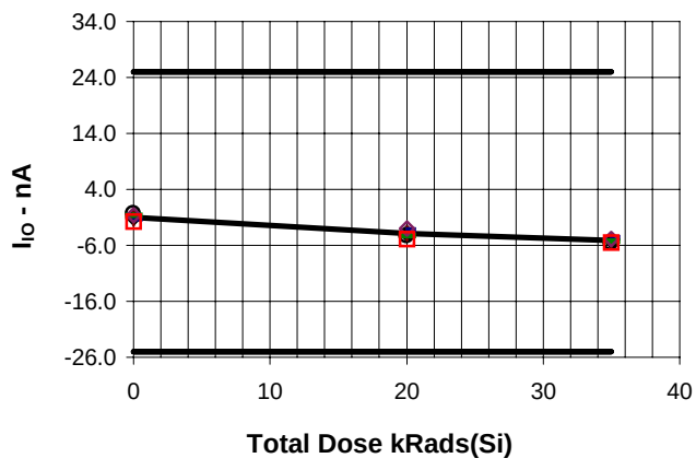
I_{IO} ; V_O=1.5V , COMP 3 vs Total Dose
