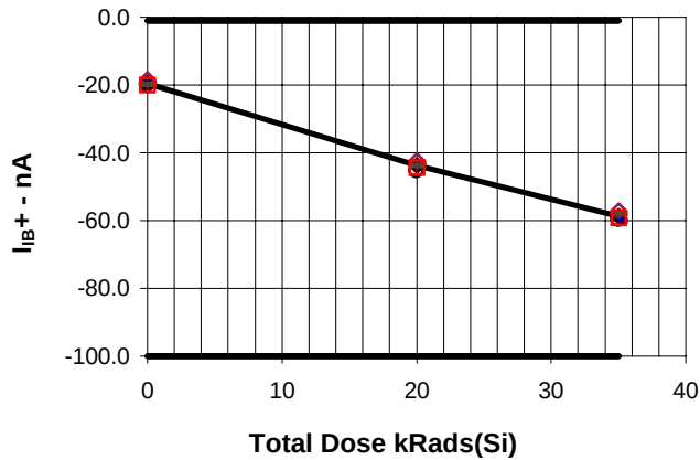
I_{B+} ; V_O=1.5V , COMP 4 vs Total Dose
