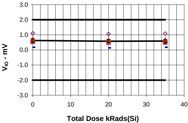
V_{IO} ; V_{CM}=28.5V , COMP 2 vs Total Dose
