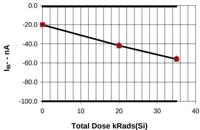
I_{IB-} ; V_O=1.5V , COMP 1 vs Total Dose
