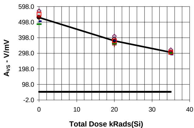
A_{VS} ; R_L=15K , COMP 4 vs Total Dose
