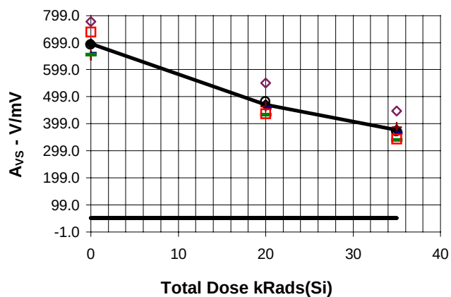
A_{VS} ; R_L=15K , COMP 3 vs Total Dose
