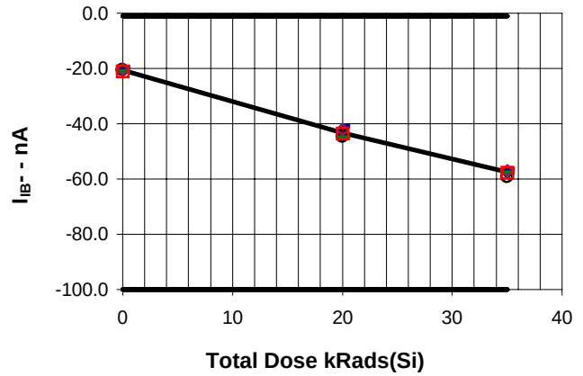
I_{B-} ; V_O=1.5V , COMP 3 vs Total Dose
