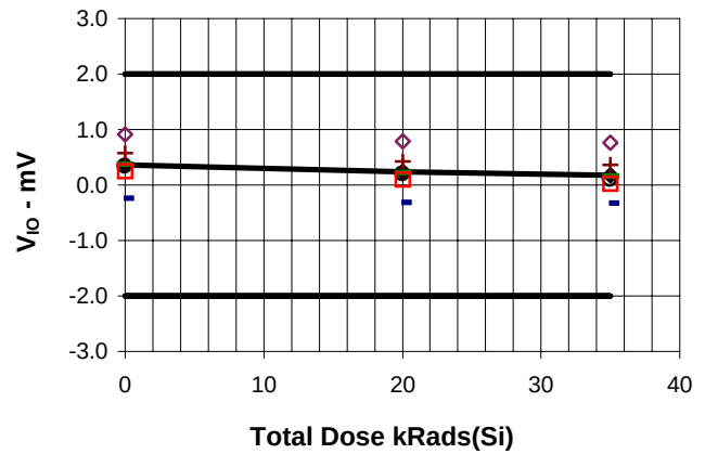
V_{IO} ; V_{+}=5V , COMP 2 vs Total Dose
