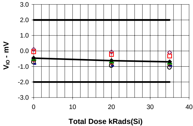
V_{IO} ; V_{+}=5V , COMP 1 vs Total Dose
