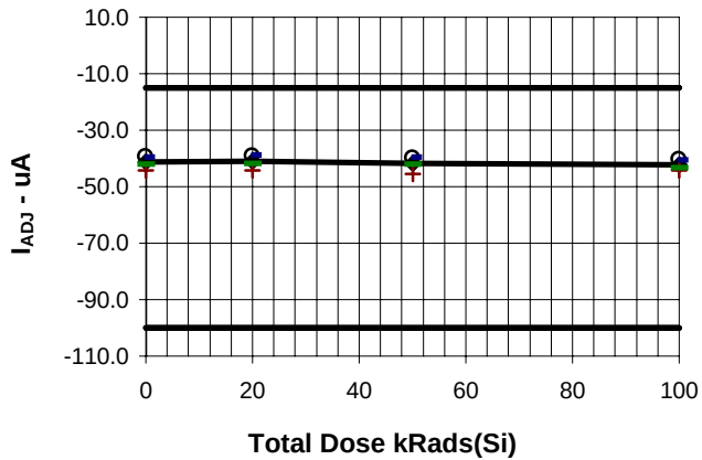
I_{ADJ} ; V_I=4.25V , I_L=-5mA vs Total Dose
