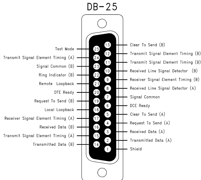
FIGURE 5. EIA/TIA-530-A DB-25
