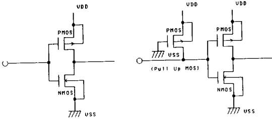
RS, R/W, RESET Terminals (Pull-Up MOS)
