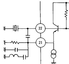
<Oscillator>
