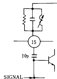
<Phase Shifter>
