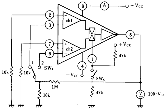
(1) I_{CC} , V_O , SVR
