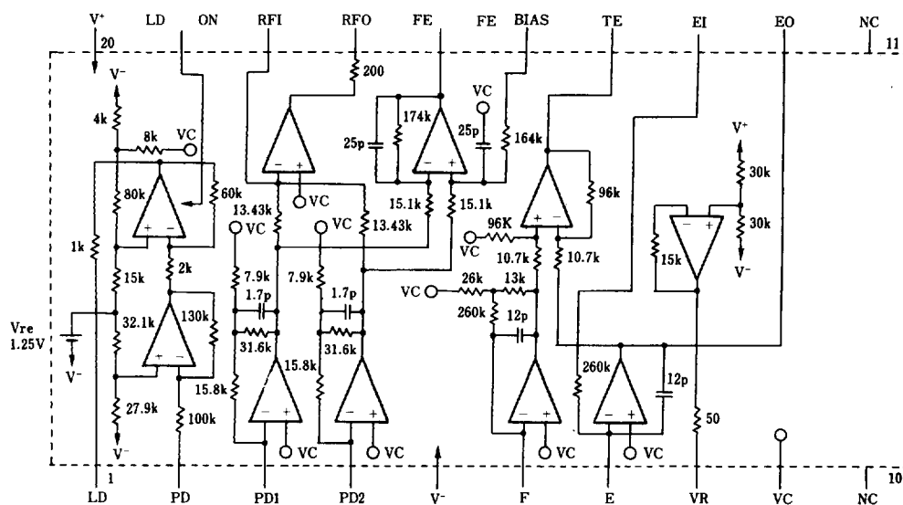
NJM2117V
