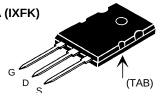
ISOPLUS 247™ (IXFR) E153432
