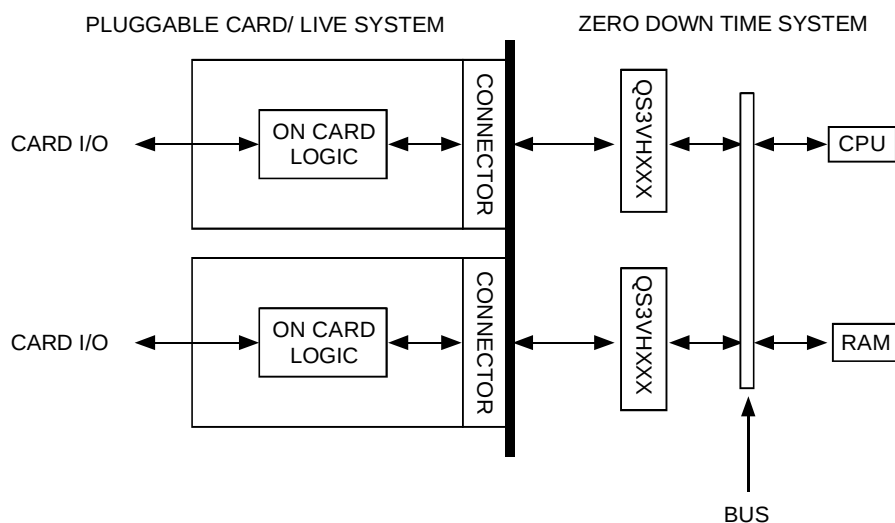
Hot Swapping
