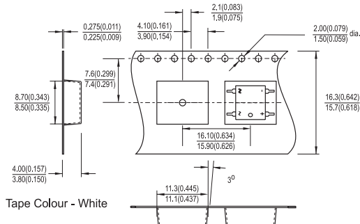
Tape Reel Dimensions for 1B...STR16/DF...STR16
