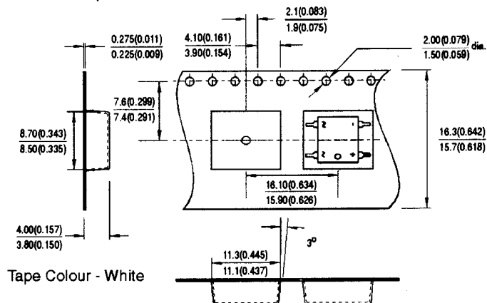
Tape Reel Dimensions for 1B...STR16/DF...STR16
